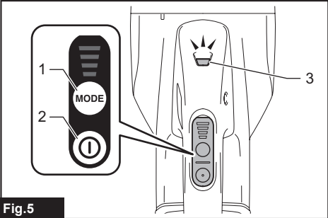
Fig.5 ► 1. Bouton de changement de la puissance d'aspiration 2. Bouton ON/OFF (marche/arrêt) 3. Lampe
